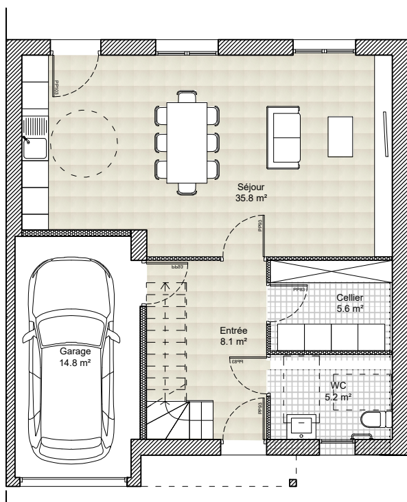
Plan Rez-de-chaussée
